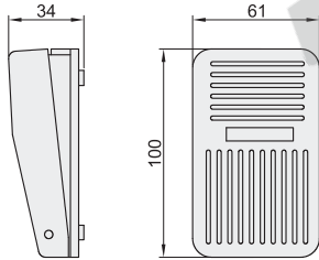
窄型 ZHB90
