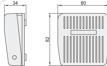
宽型 ZHB91
