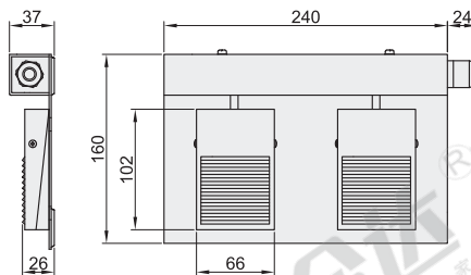
双脚踏 ZHB94
