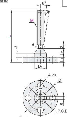
法兰底座型 TBD32
