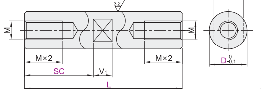
带扳手槽型 RAD11/12/13/16/18
