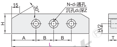
ZD(侧面沉孔)
