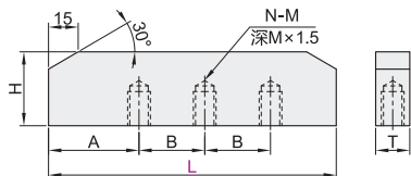
ZB(底面螺孔)
