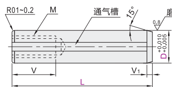
带通气槽型·公差p6
