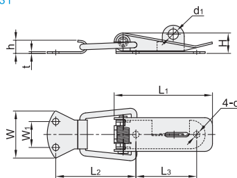
安装孔孔距
