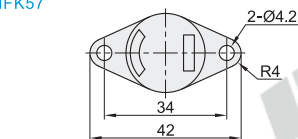
顺时针阻尼型 HFK57
