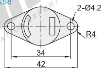
逆时针阻尼型 HFK58
