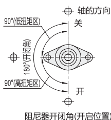
阻尼器开闭角(开启位置)
