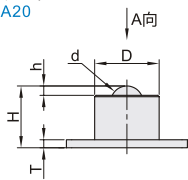
方法兰式 QDA20
