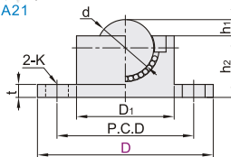
圆法兰式 QDA21
