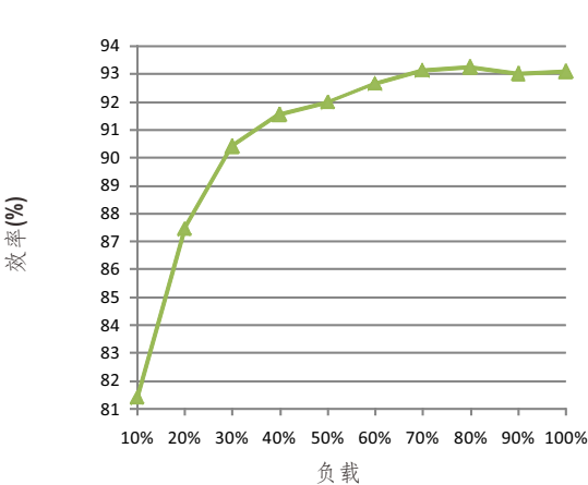
效率vs负载(48V机型)
