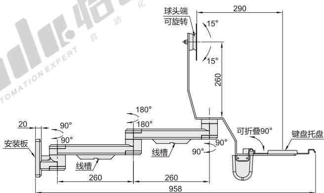
键盘托盘尺寸
