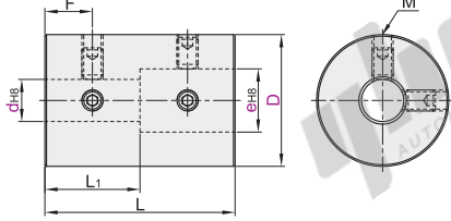
螺钉固定型 DCP11
