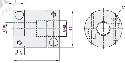
螺钉夹紧型 DCP12
