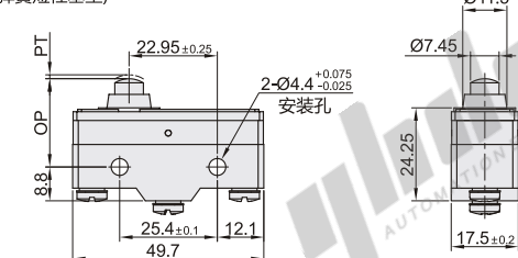
1(弹簧短柱塞型)
