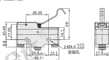
H(带弯曲摆杆型)
