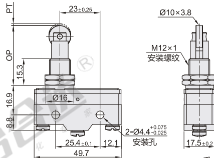
L(小竖轮柱塞型)
