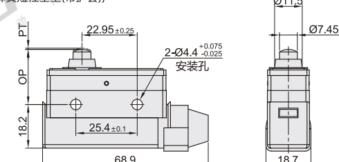
N(彈簧短柱塞型(帶护套))
