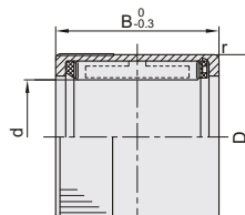
树脂簧片·带滚花 HF...-KF-R
