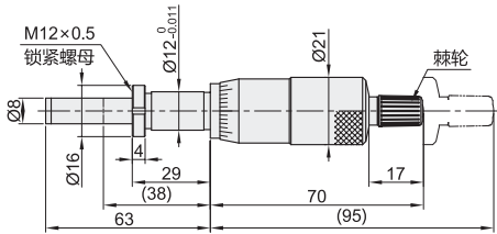
带锁紧螺母·平面测量面 EPF06-151-223
