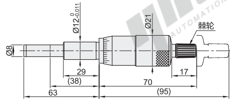
直柄型·平面测量面 EPF06-151-224
