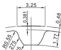
标准齿形
