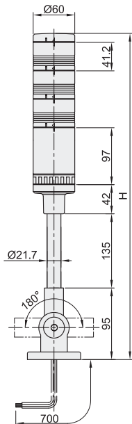
A(可折式)
