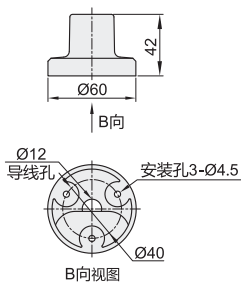
B向视图
