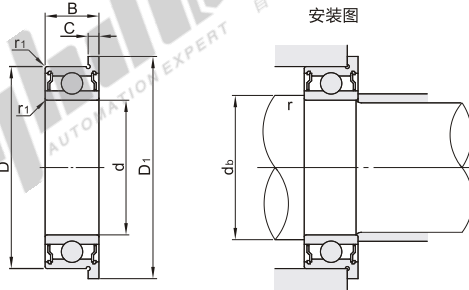
安装图
