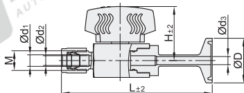
卡套+快装 XLA06
