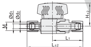
两端卡套 XLA05
