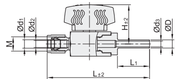
卡套+焊接 XLA07
