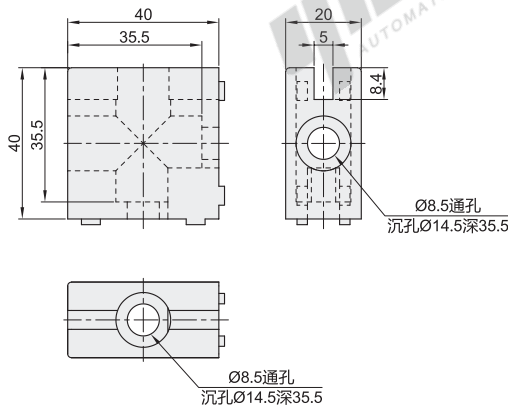
门滑槽固定块 AMS51-C AMS53-C
