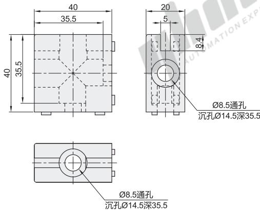
门滑槽固定块 AMS51-C AMS53-C
