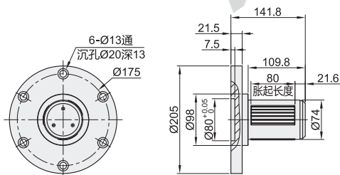
齿片式单头 ZCF41/44/47
