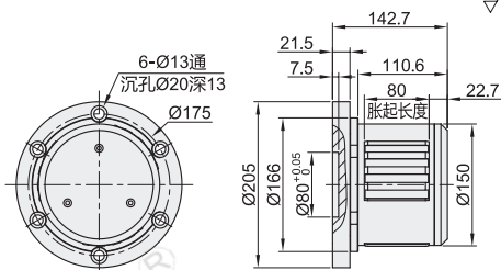
齿片式单头 ZCF41/44/47
