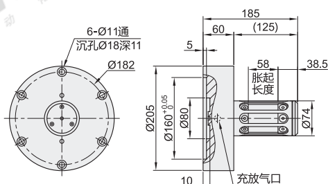
键式单头 ZCF43/46/49
