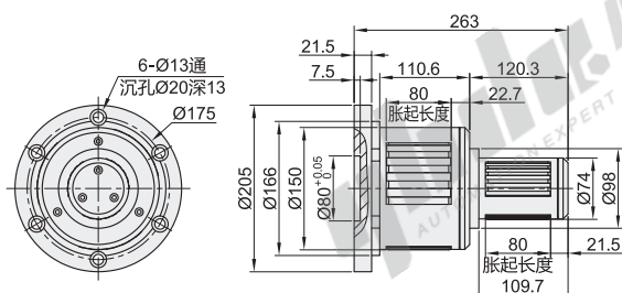
齿片式双头 ZCF42/45/48
