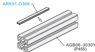
分解图
