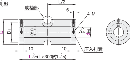
带肋槽直柱型 ENF21/26/31
