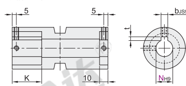
键槽孔+螺孔型
