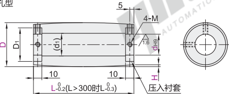
带肋槽直柱型 ENF21/26/31
