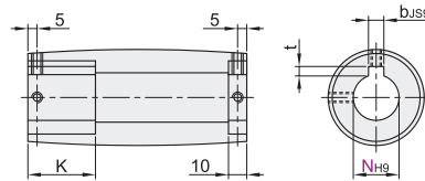
键槽孔+螺孔型
