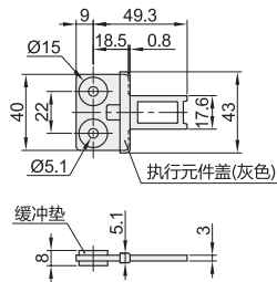
1系列·直线型·附缓冲垫 XBS10-1-A-X
