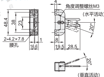
5系列·水平/垂直活动型·附缓冲垫 XBS10-5-D-X
