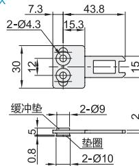
5系列·直线型·附缓冲垫 XBS10-5-A-X
