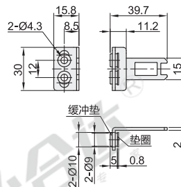
5系列·水平/垂直活动型·附缓冲垫 XBS10-5-D-X
