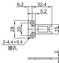
5系列·直线型 XBS10-5-A
