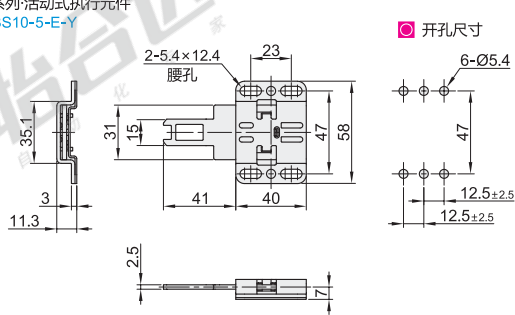
5系列·活动式执行元件 XBS10-5-E-Y
