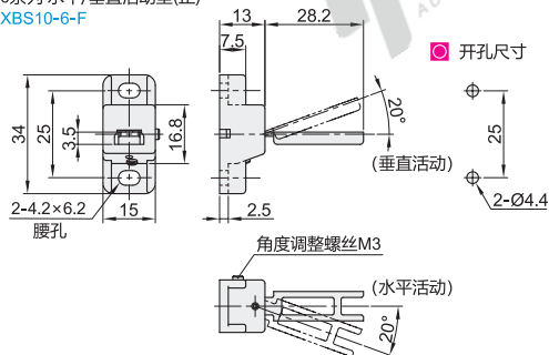
6系列·水平/垂直活动型(正) XBS10-6-F
