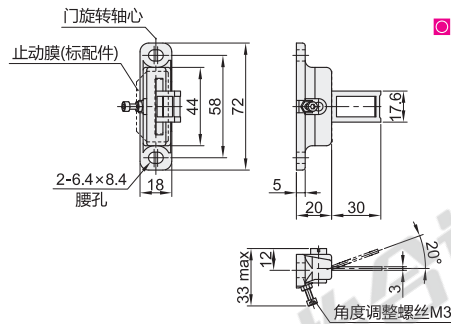
5系列·直线型·附缓冲垫 XBS10-5-A-X
