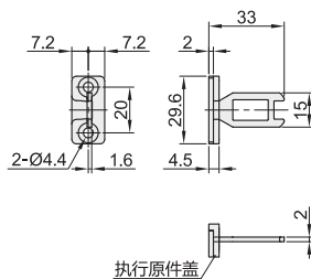
5系列·L型 XBS10-5-B
