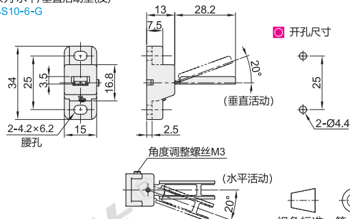
6系列·水平/垂直活动型(反) XBS10-6-G
