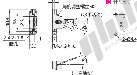
5系列·水平/垂直活动型 XBS10-5-D
