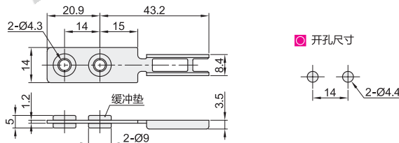
6系列·L型·附缓冲垫/固定板 XBS10-6-B-Z
