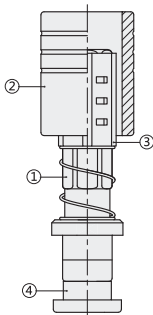
无挡块 OGH41
