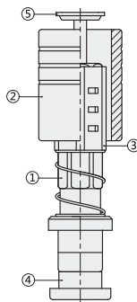
弹簧
