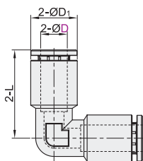
弯接头 XZS63
