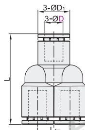
Y型三通接头 XZS65
