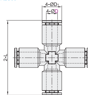
十字四通接头 XZS66
