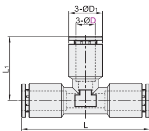
T型三通接头 XZS64
