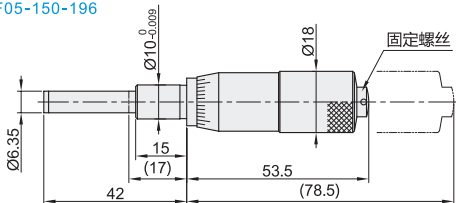
直柄型·平面测量面 EPF05-150-196
