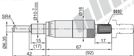
直柄型·球面测量面 EPF04-150-801
