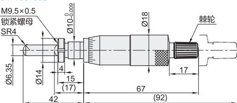
带锁紧螺母·平面测量面 EPF05-150-195
