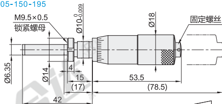
带锁紧螺母·平面测量面 EPF05-150-195
