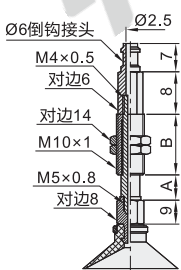
盘径 \varnothing 10\sim 16
