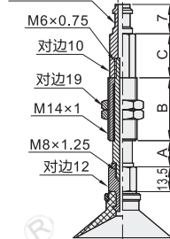
盘径 \varnothing 40, \varnothing 50
