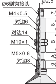
盘径 \varnothing 20\sim 32
