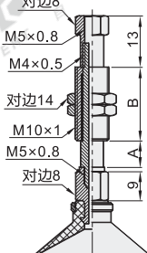
盘径 \varnothing 20\sim 32
