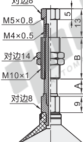
盘径 \varnothing 10\sim 16
