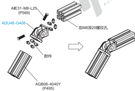
分解图
