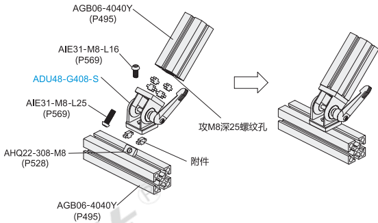
分解图
