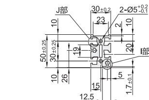
型材截面放大图
