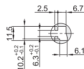
J部(M6用)
