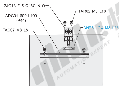
分解图
