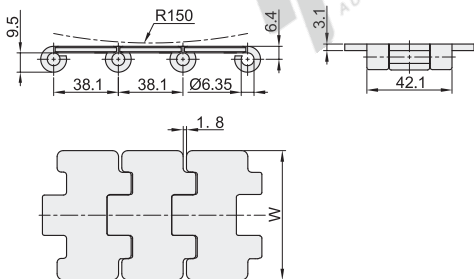
链条-单铰链 VMX51
