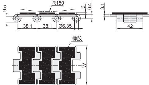
链条-单铰链防滑型 VMX52
