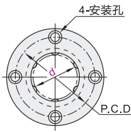
圆法兰型
