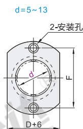
对边法兰型
