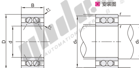
安装图
