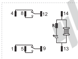
☑ ZHY05接线图
