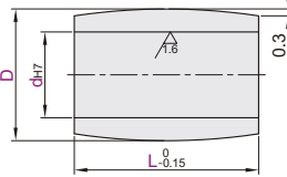
圆弧形 QAQ21/22
