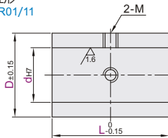
直柱形 QAR01/11
