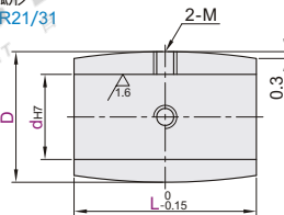
圆弧形 QAR21/31
