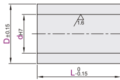
直柱形 QAQ01/02/11/12
