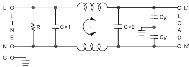
配线图
