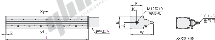
X-X剖面图
