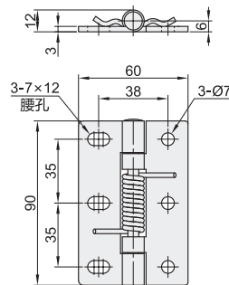
圆孔+腰孔型 HFG52
