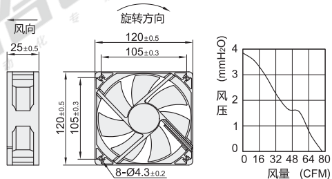
外形尺寸: 120B
