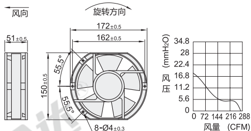
外形尺寸: 17251M2
