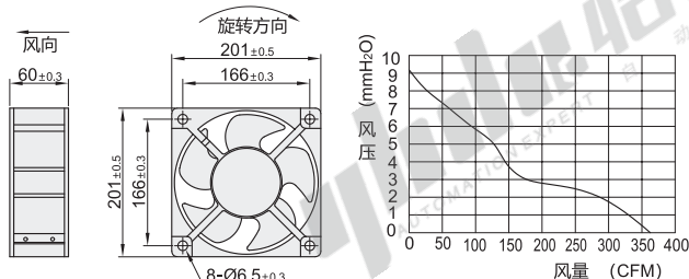
外形尺寸: 20060M2
