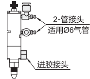
装配示意图
