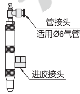
装配示意图
