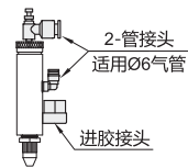
装配示意图
