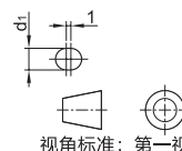
定位腰孔尺寸图
