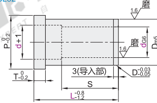
无油槽 OGL52
