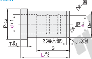
有油槽 OGL51
