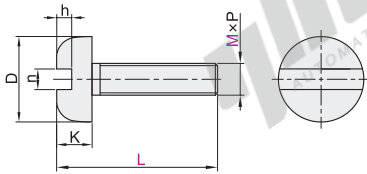
一字槽盘头螺钉 TAP25
