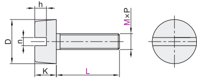
一字槽圆柱头螺钉 TAP31
