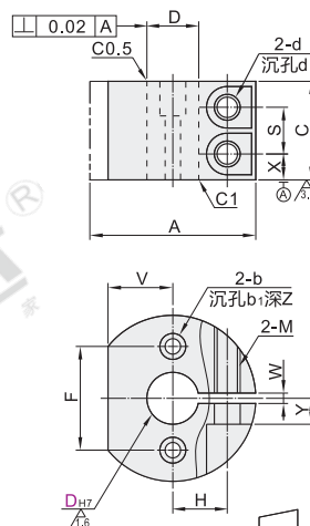
沉孔型 RCP21/22
