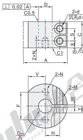
螺孔型 RCP11/12/16
