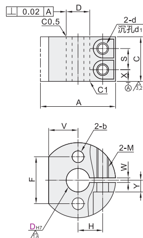
通孔型 RCP01/02/06/08
