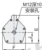
X-X剖面图
