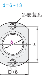
对边法兰型 Y-J-GVC51/52
