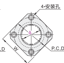
方法兰型 Y-J-GVC41/42
