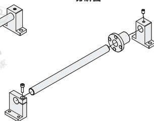
分解图
