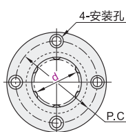
圆法兰型 Y-J-GVC31/32
