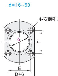
对边法兰型 Y-J-GVC51/52
