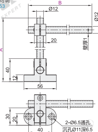
双管可调 ZLP53
