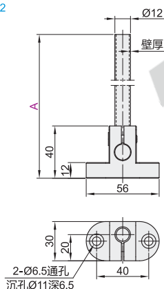
三管可调 ZLP54
