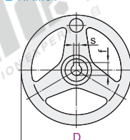
键槽孔型 E-HAM01
