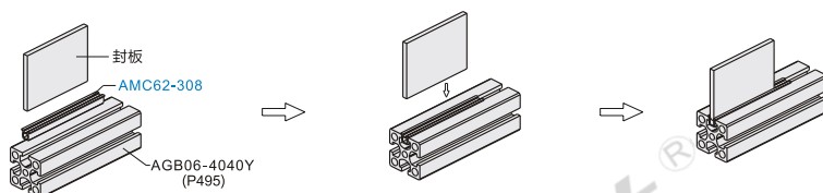
分解图
