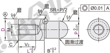
小头内螺纹型 YPV61/66
