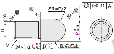
大头外螺纹型 YPV21/26
